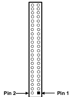
IDE1 Header
